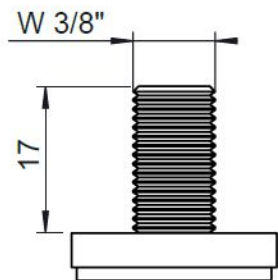
TERMINAL TIPO T/M ROSCA EXTERNA (PARAFUSO)
